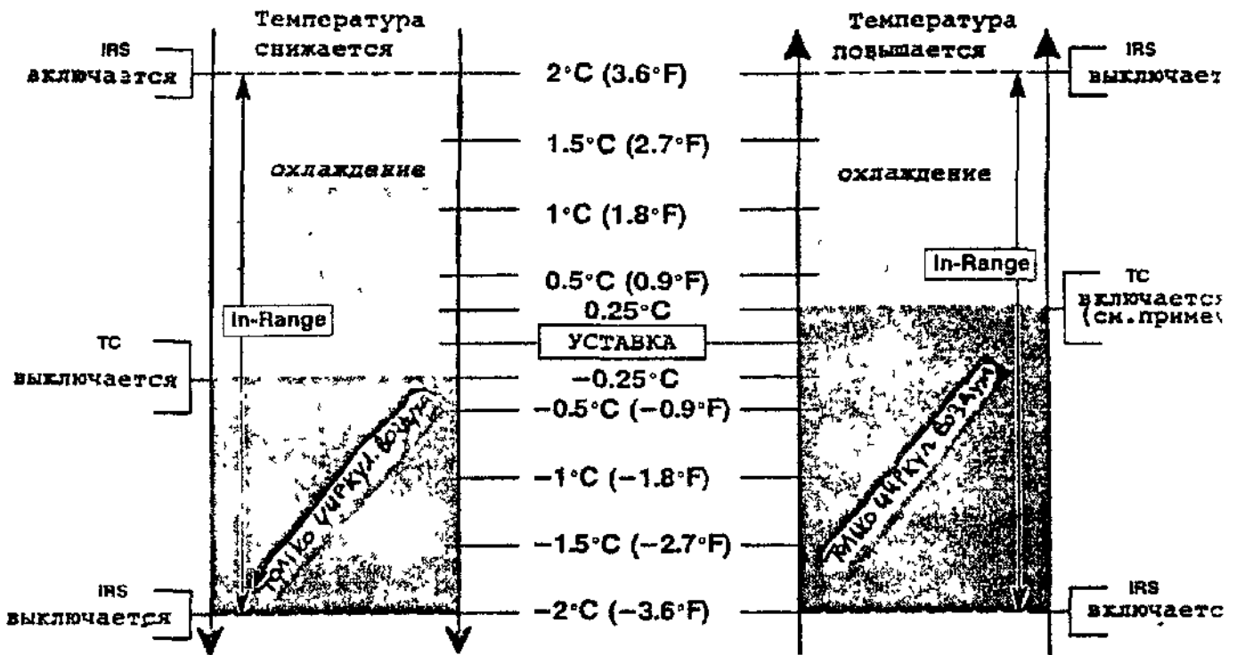
Рис.1.9 Контрольное у-во настроено ниже -10°C (14°F) - Контроль обратного воздуха
